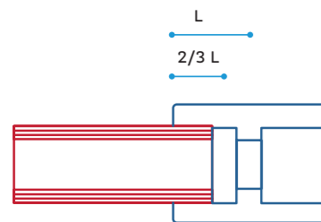
Figura 6. Termofusión a socket.
