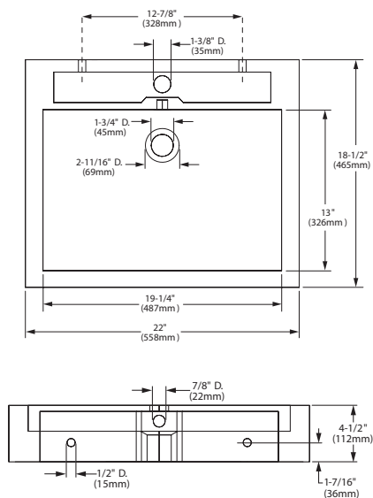
Perforación para monomando 0621001.020 Blanco ○ Lavabo de sobreponer Studio 22
