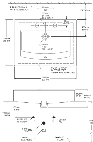
Perforación para monomando 0504001.020 Blanco ○ Lavabo de sobreponer Boxe
